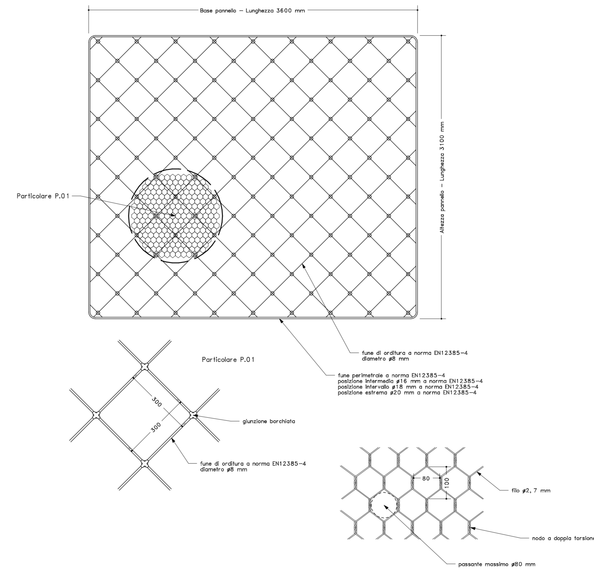
VISTA IN SEZIONE E DALL'ALTO FERMANEVE
