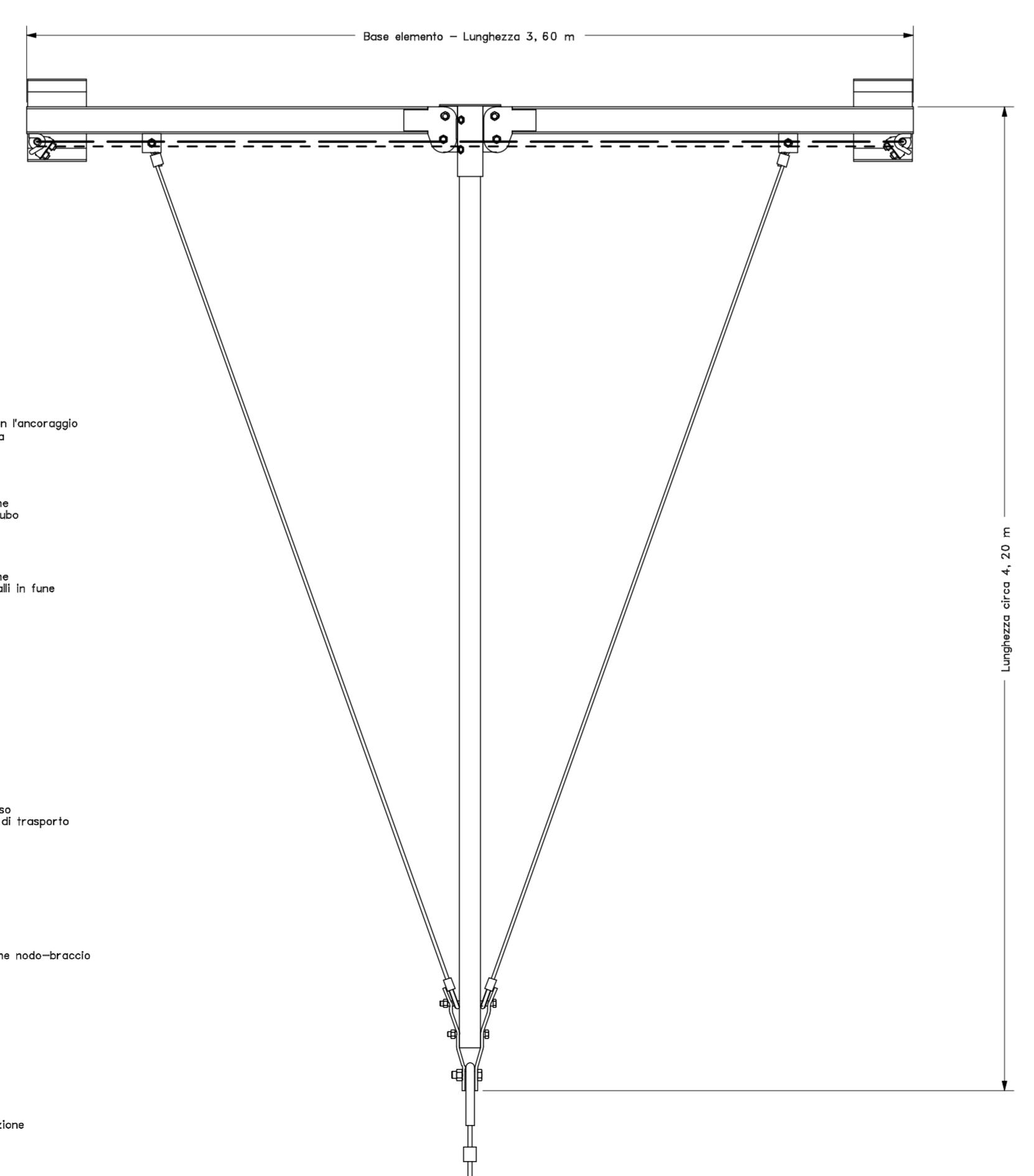
VISTA DALL'ALTO FERMANEVE
