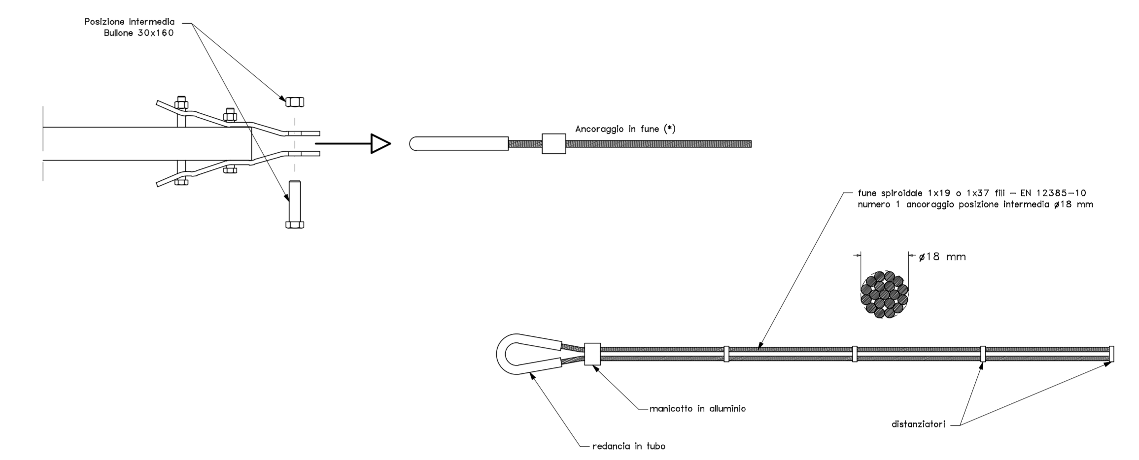
PARTICOLARE CONNESSIONE AL PUNTO DI ANCORAGGIO
