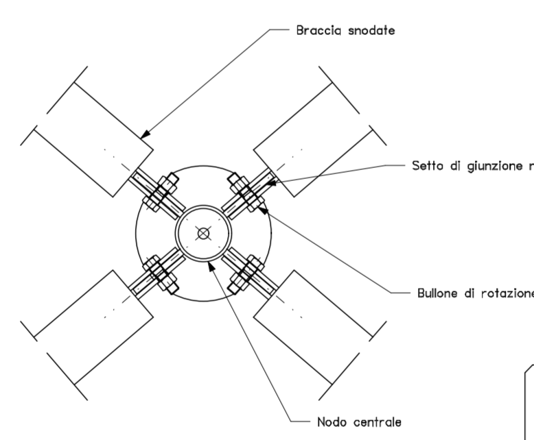
Particolare P.02 / Vista Laterale
