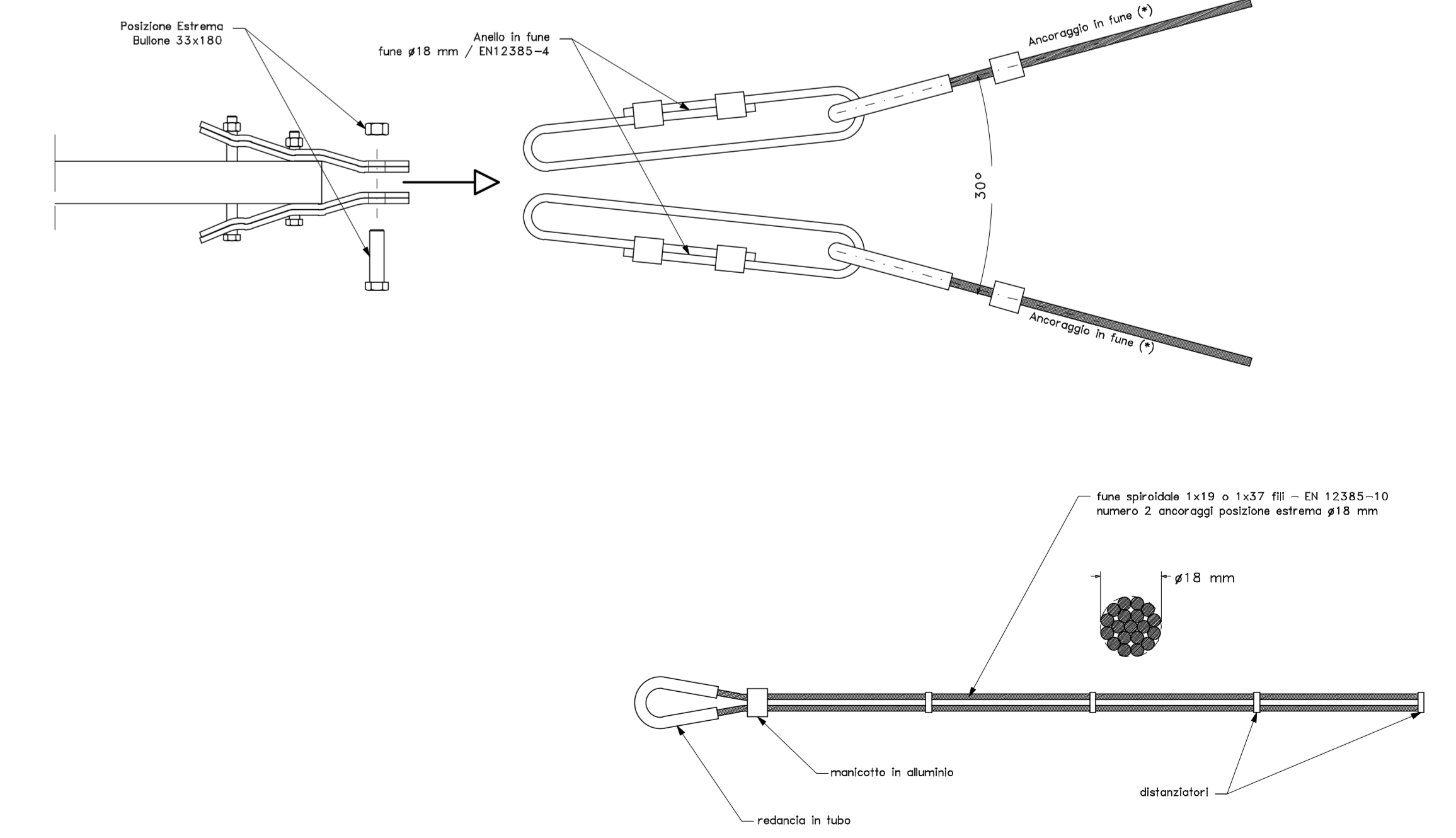
PARTICOLARE CONNESSIONE AL PUNTO DI ANCORAGGIO
