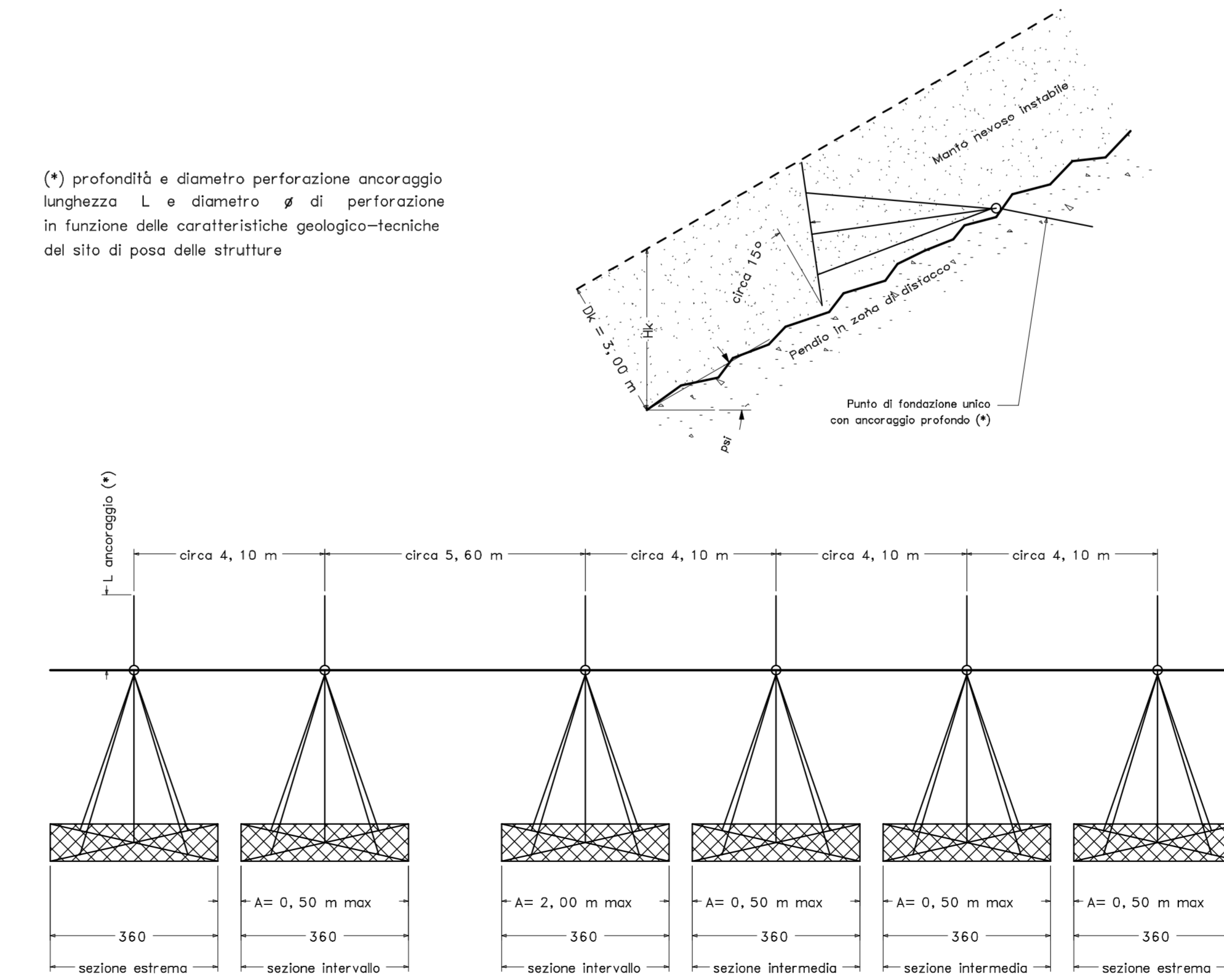
PARTICOLARE CONNESSIONE AL PUNTO DI ANCORAGGIO
