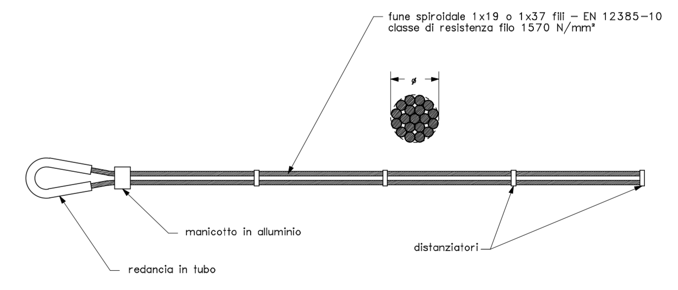
ANCORAGGIO IN FUNE SPIROIDALE
