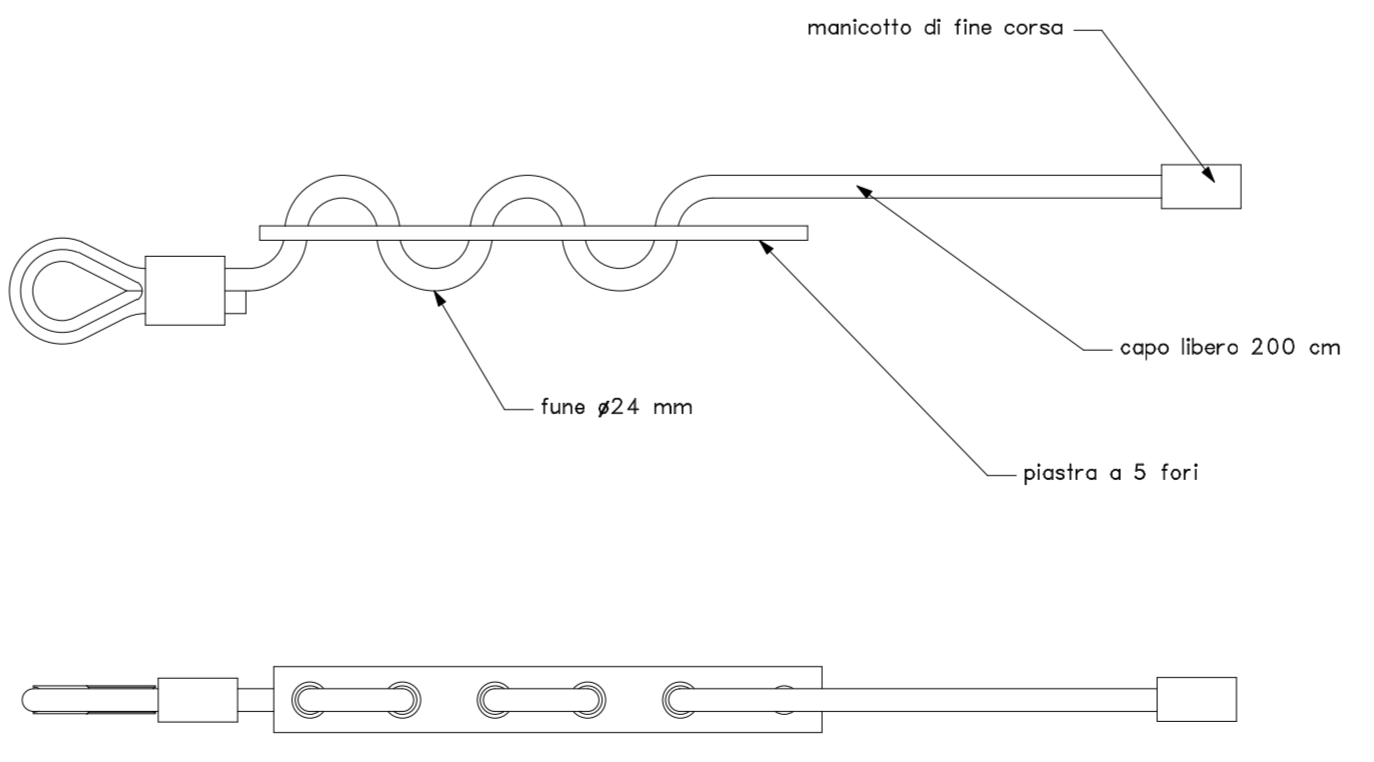
SISTEMA FRENANTE #24 mm / 200 kJ
