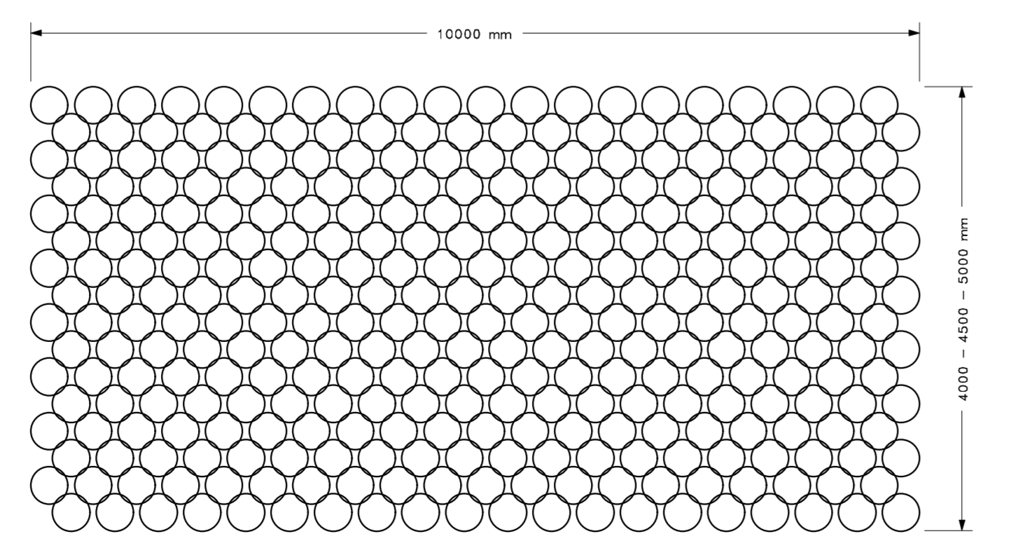
PARTICOLARE PANNELLO AD ANELLI CONCATENATI anelli in fune EN 12385-10 #10, 5 / #350 mm
