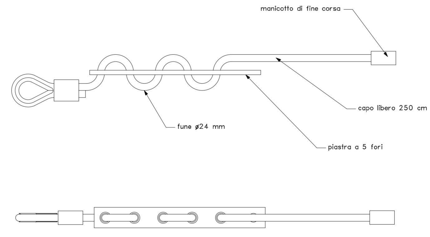
SISTEMA FRENANTE #24 mm / 250 kJ
